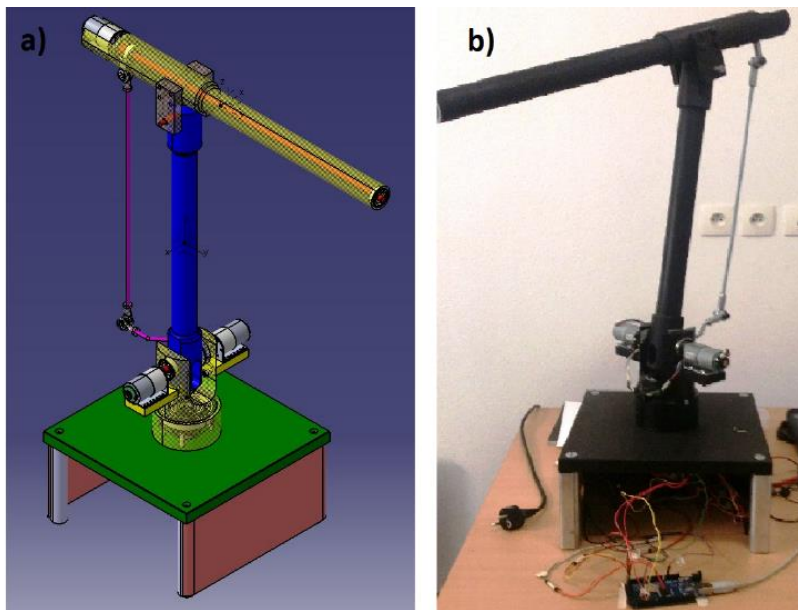
Figura 1. a) Esquema de robot manipulador de mecanismo de 5 barras, realizado en software CATIA V5, y b) Robot manipulador manufacturado a partir del esquema de diseño mecánico.
